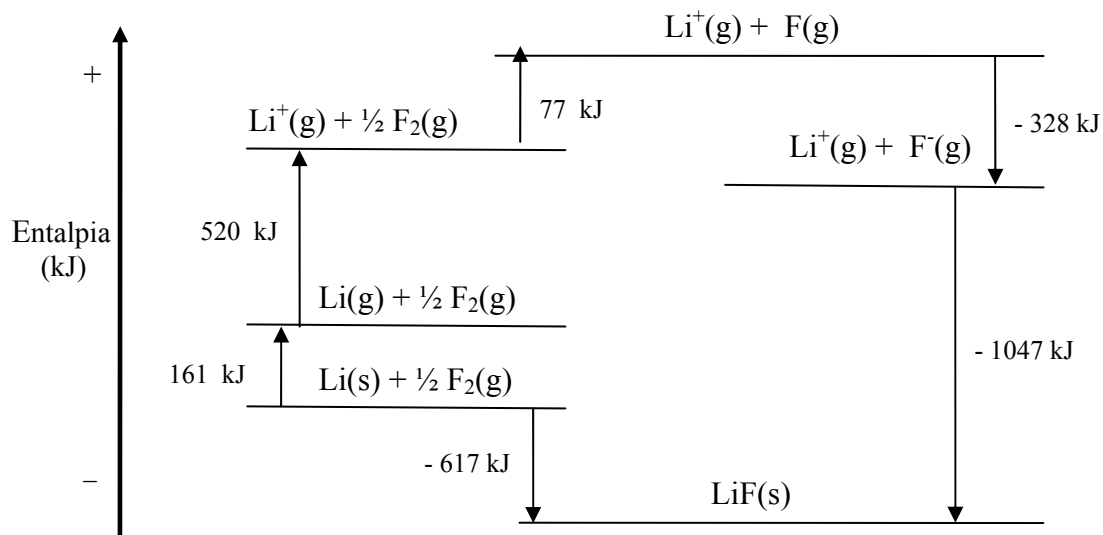
Diagrama d'entalpies del fluorur de liti
